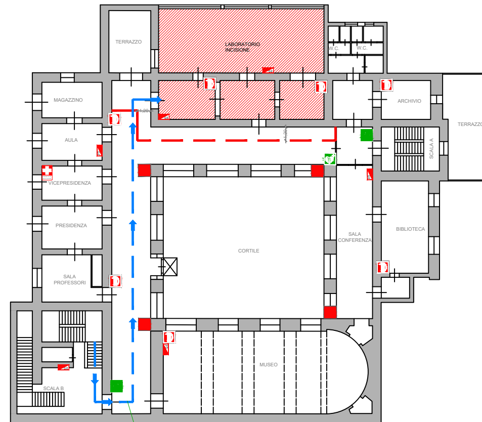
PIANO PRIMO
